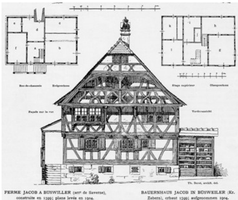
Exemple : Ferme Jacob de Buswiller construite en 1599. Plans levés en 1904.
